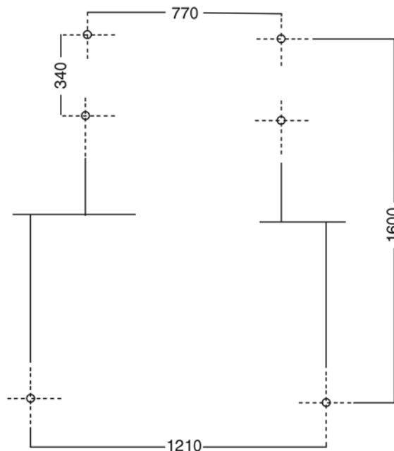
ΣΧΕΔΙΟ ΕΓΚΑΤΑΣΤΑΣΗΣ ΒΑΣΗΣ ΗΛΙΑΚΟΥ SIEMENS 130 LX
