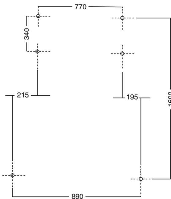
ΣΧΕΔΙΟ ΕΓΚΑΤΑΣΤΑΣΗΣ ΒΑΣΗΣ ΗΛΙΑΚΟΥ SIELINE 120 SX
